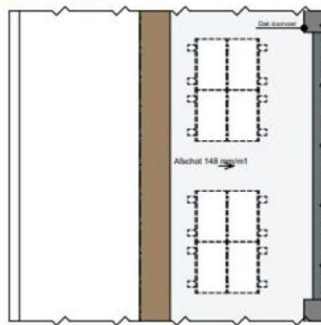
DAKOVERZICHT
