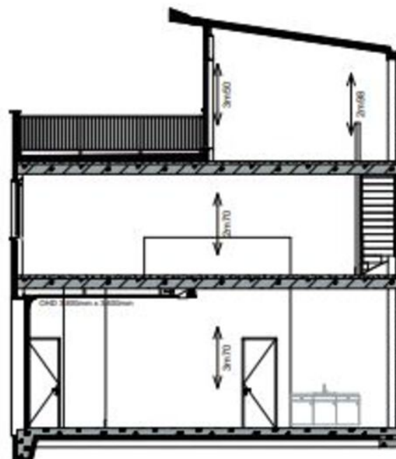
PRINCIPE DOORSNEDE
