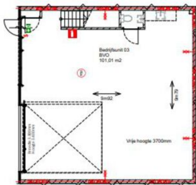
BEGANE GROND
