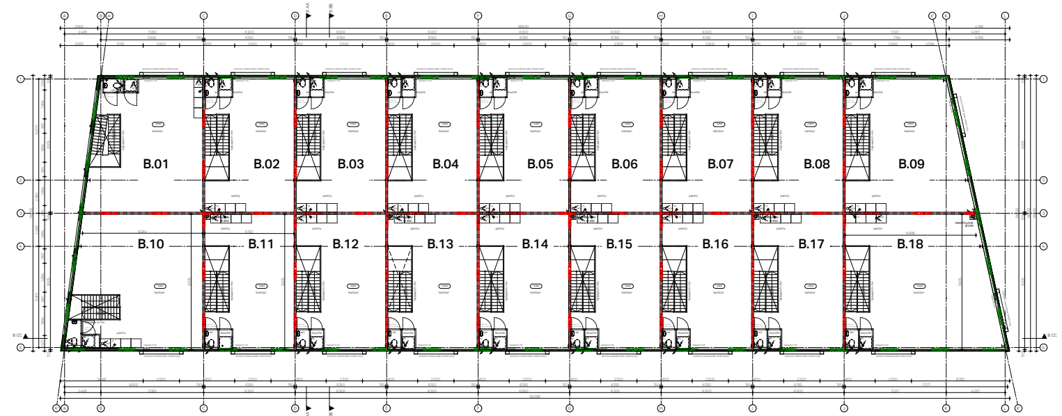
Eerste verdieping +5600 Gebouw B
