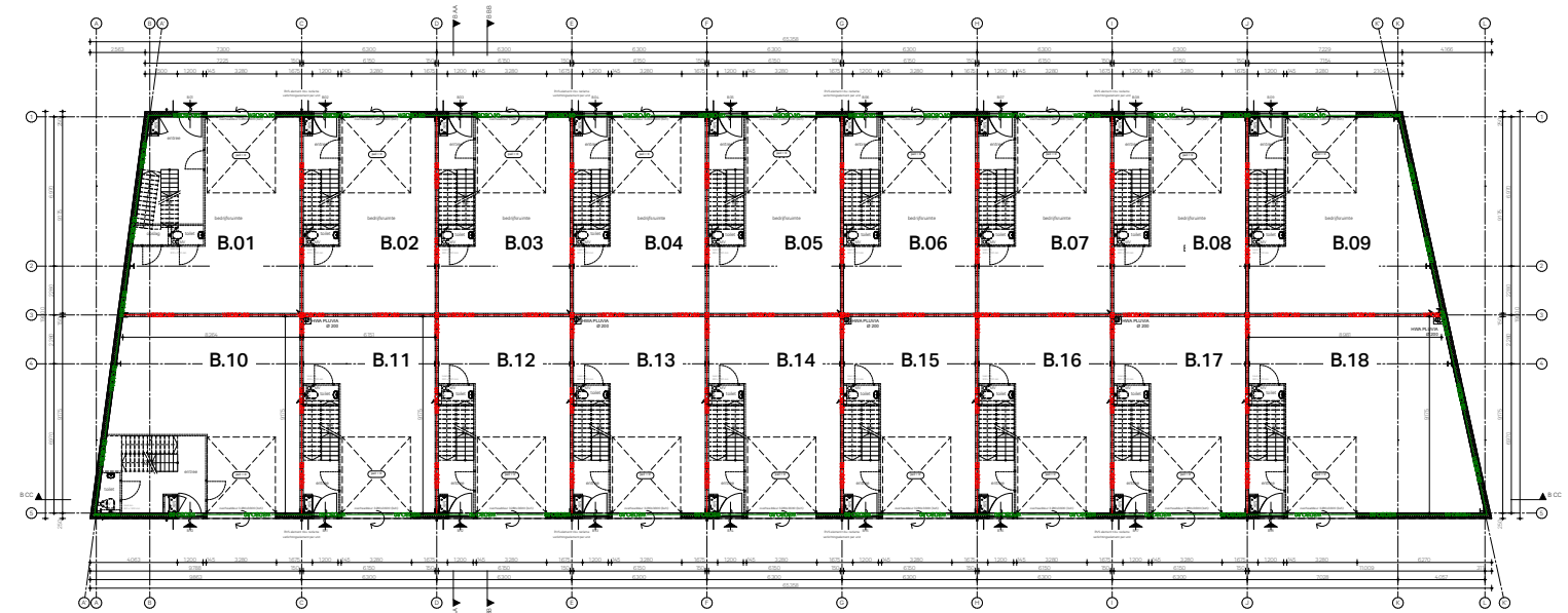
Begane grond Gebouw B
