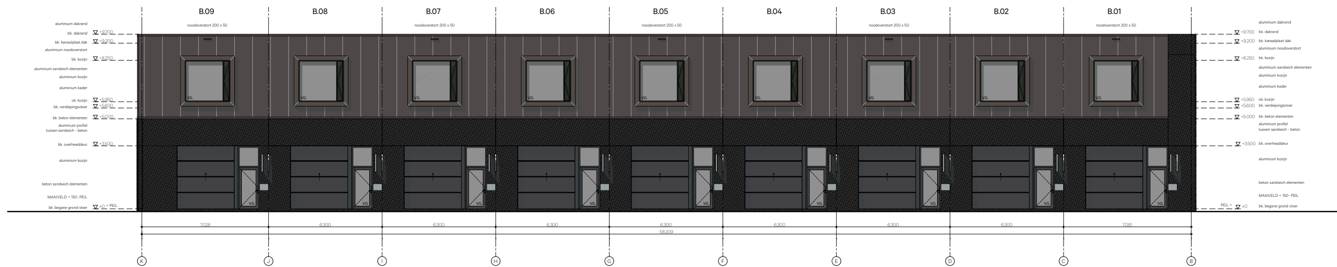
Noordgevel Gebouw B
